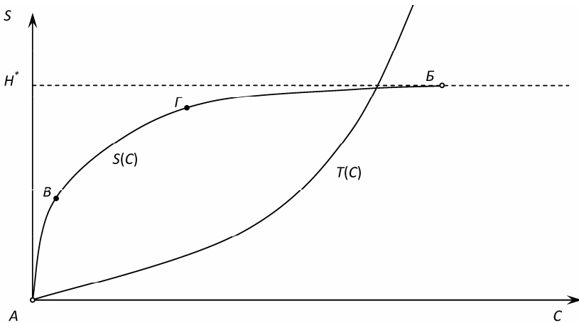
Рис. 2. Зависимость пропускной способности канала S от величины информационных затрат C Штриховая прямая H^* отражает теоретический максимум пропускной способности (8)
